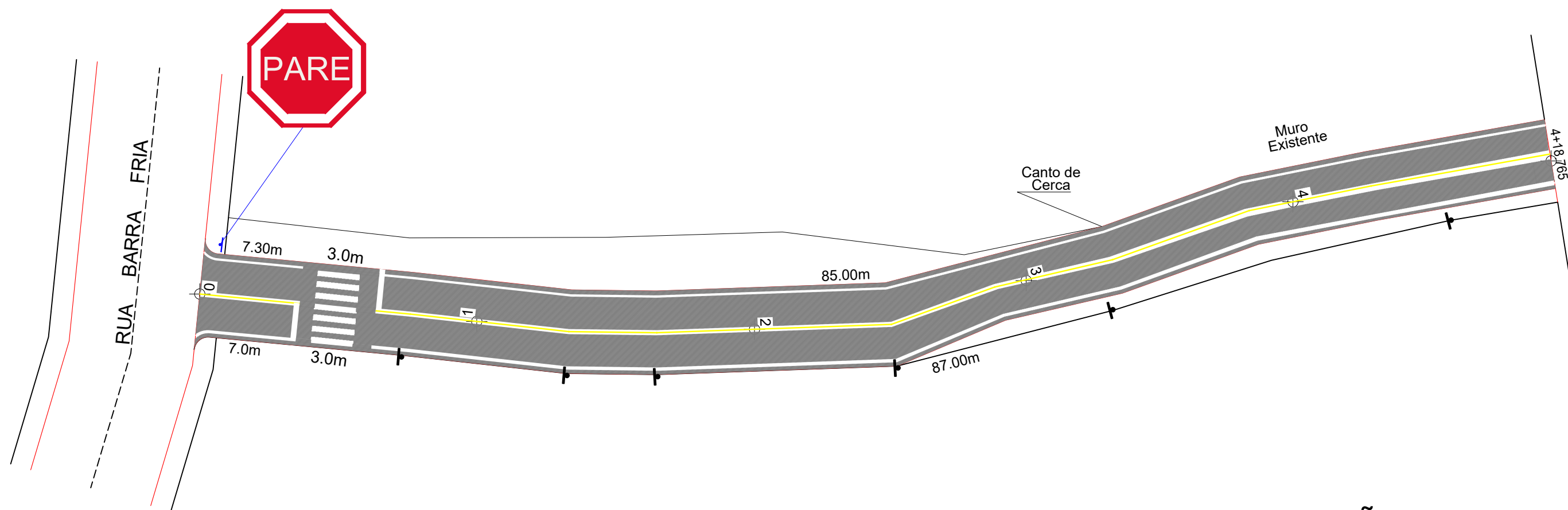
PLANTA DA SINALIZAÇÃO DA RUA ESCALA: 1/500
