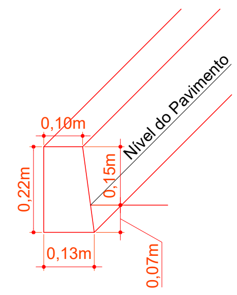
DETALHE MEIO FIO MOLDADO IN LOCO EXTRUSADO ESCALA: 1/10
