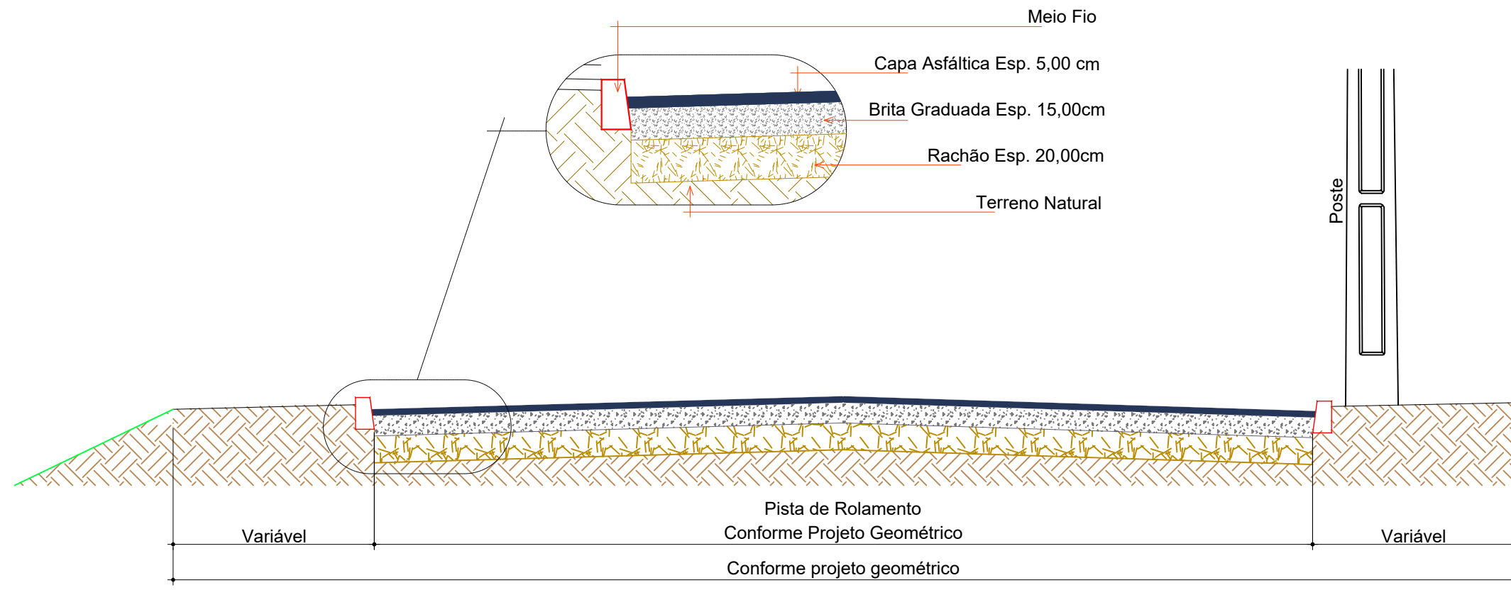
SEÇÃO TRANSVERSAL ESCALA: 1/40
