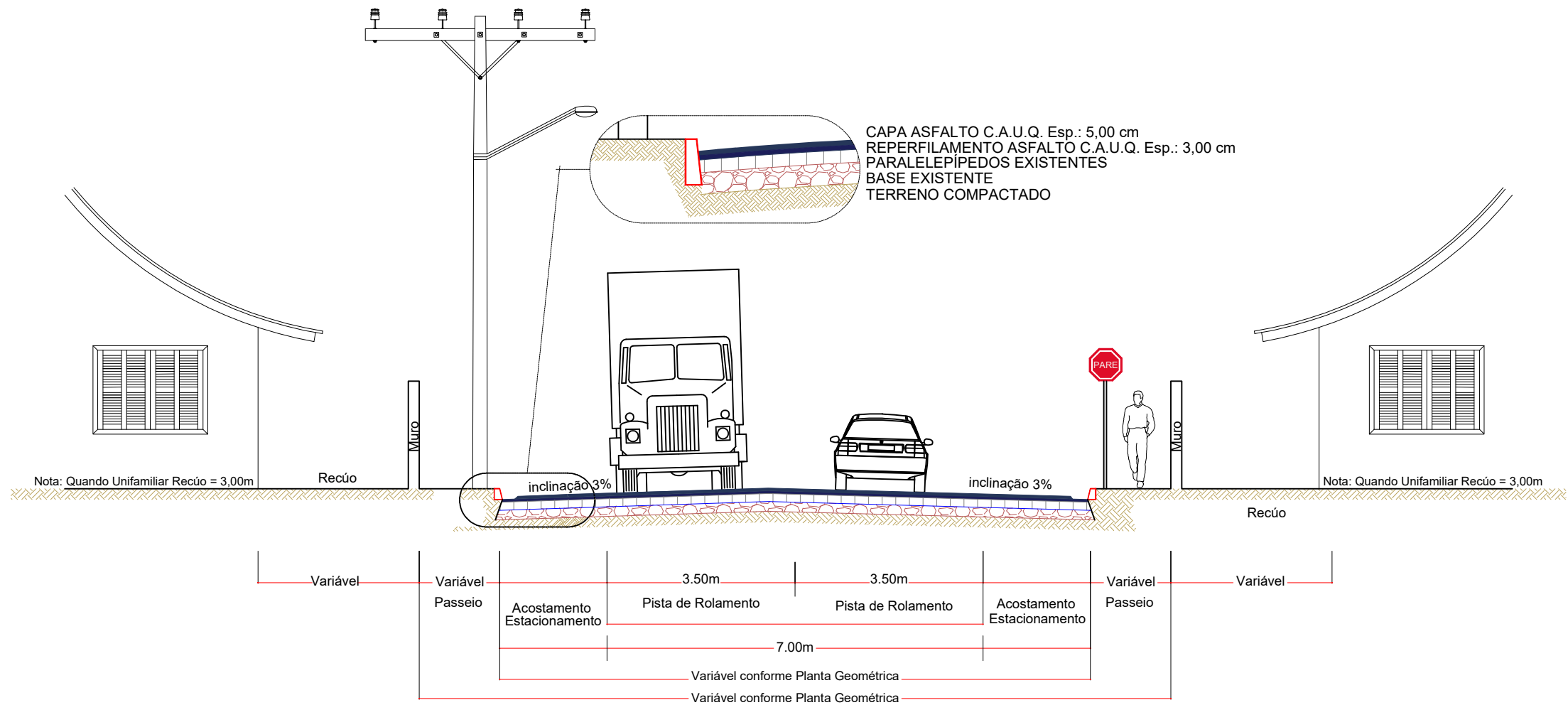
SEÇÃO TRANSVERSAL ESCALA: 1/750
