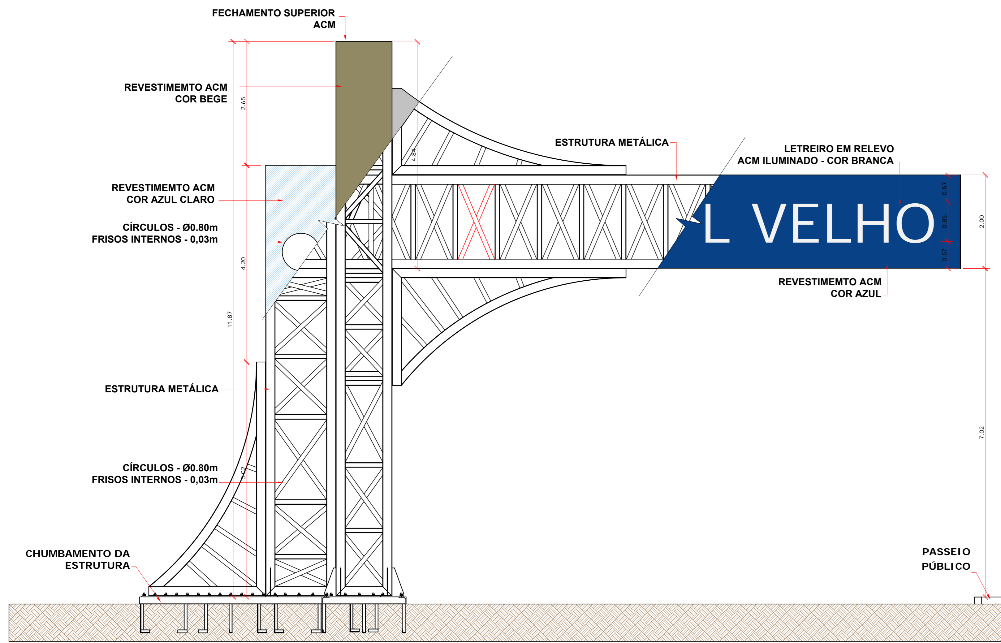
CORTE ESQUEMÁTICO (MAIORES DETALHES VER PROJETO MECÂNICO) ESCALA = 1 : 50
