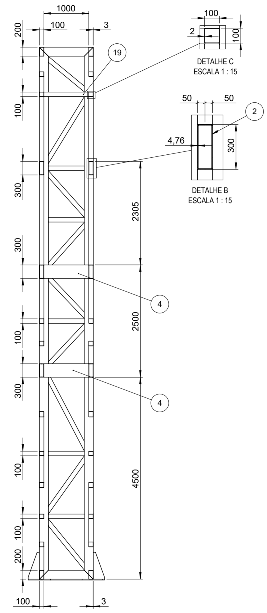
SEÇÃO A-A
