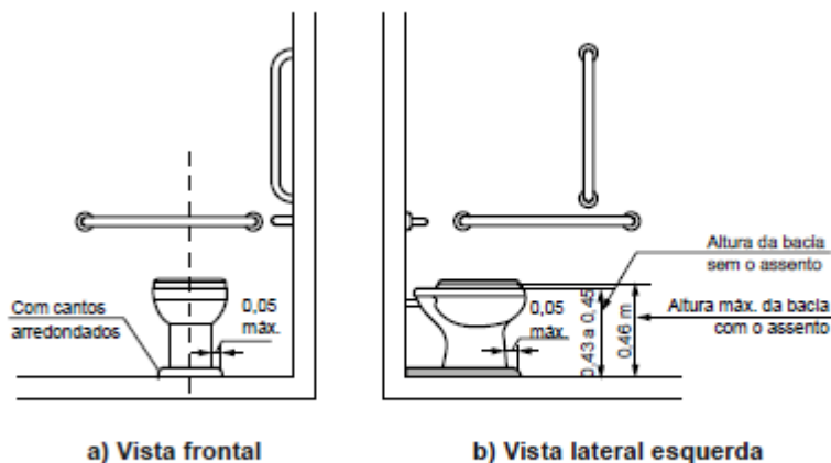
Figura 104 – Bacia com sóculo
