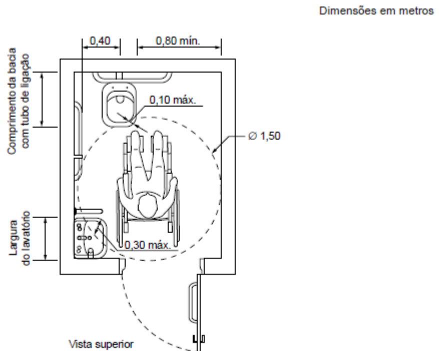
Figura 99 – Medidas mínimas de um sanitário acessível
