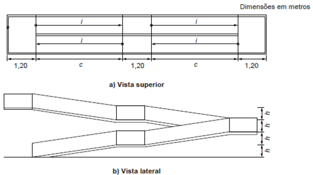
Figura 70 – Dimensionamento de rampas
