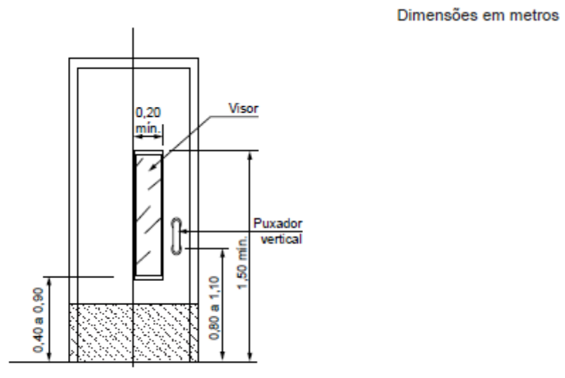
Figura 85 – Porta do tipo vaivém
