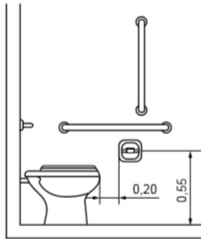
Figura 123 – Localização da papelaria embutida – Vista lateral
