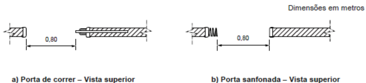
Figura 83 – Vãos de portas de correr e sanfonada
