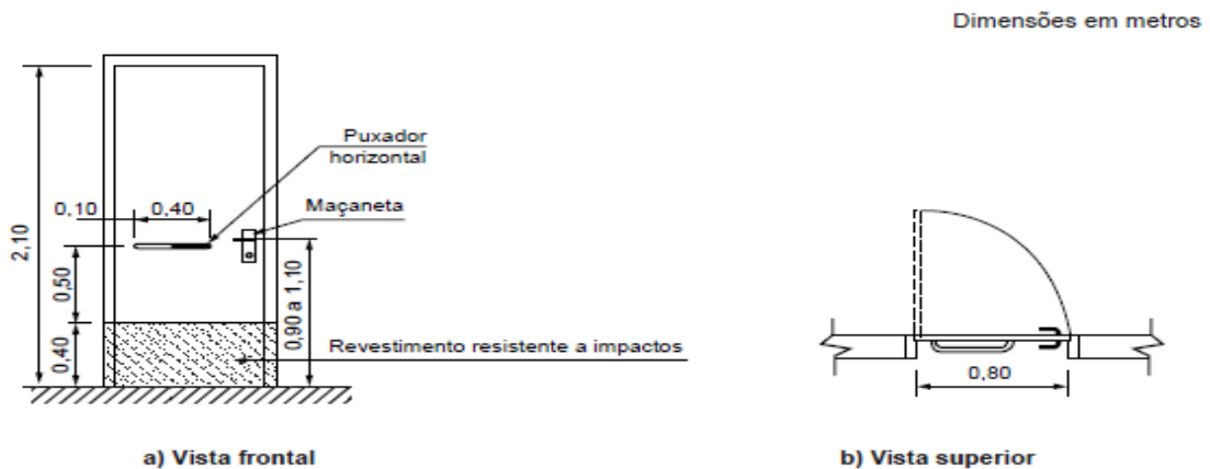
Figura 84 – Portas com revestimento e puxador horizontal
