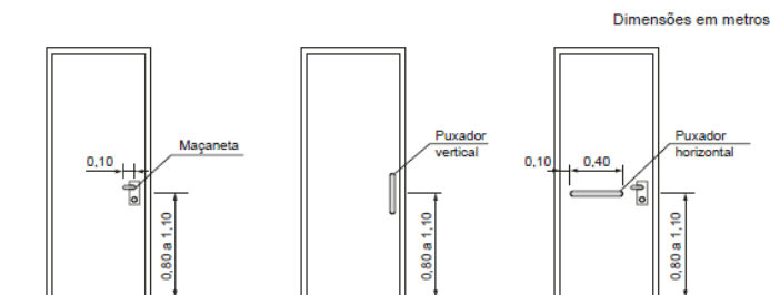
Figura 20 – Maçanetas e puxadores – Exemplos
