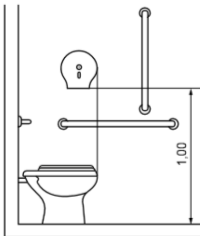
Figura 124 – Localização da papelaria de sobrepor (rolo) – Vista lateral
