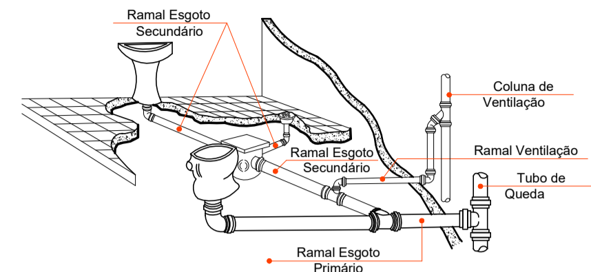
DETALHE COLUNA DE VENTILAÇÃO
