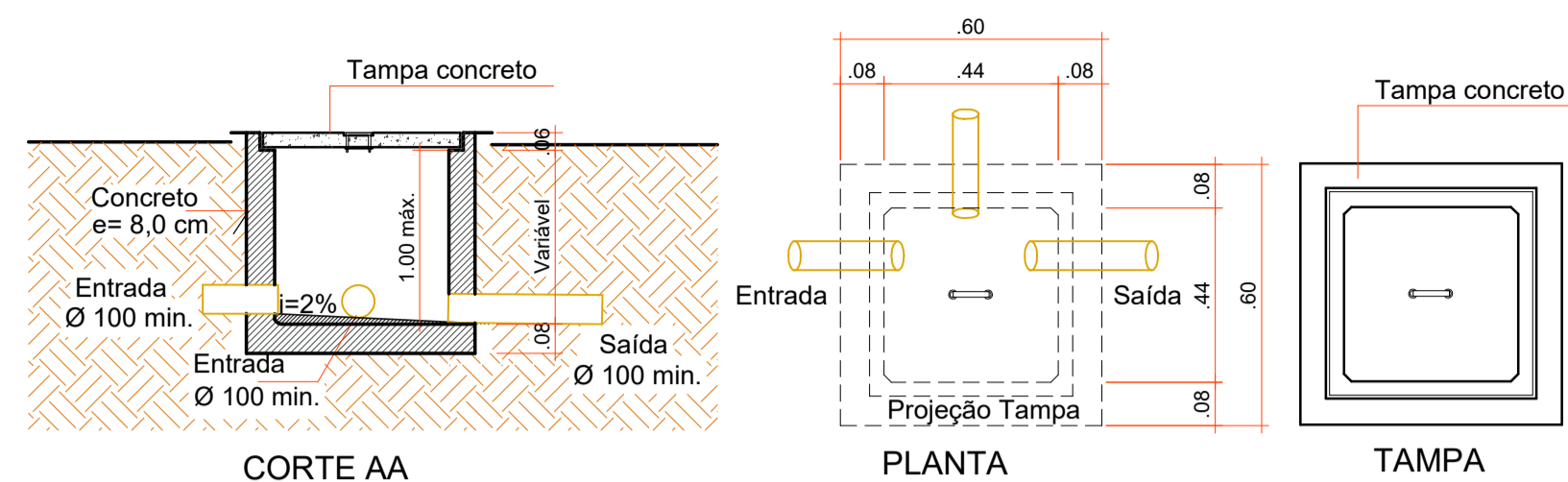
DETALHE CAIXA DE INSPEÇÃO
