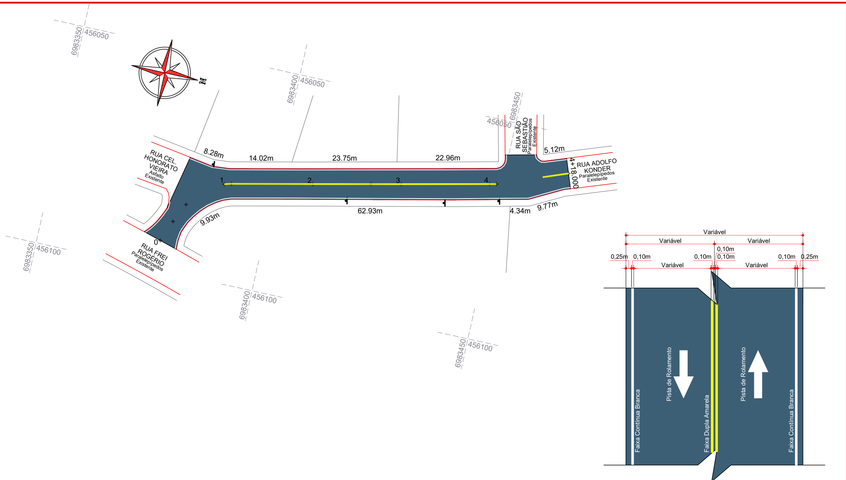
DETALHE DA SINALIZAÇÃO HORIZONTAL ESCALA: 1/100
