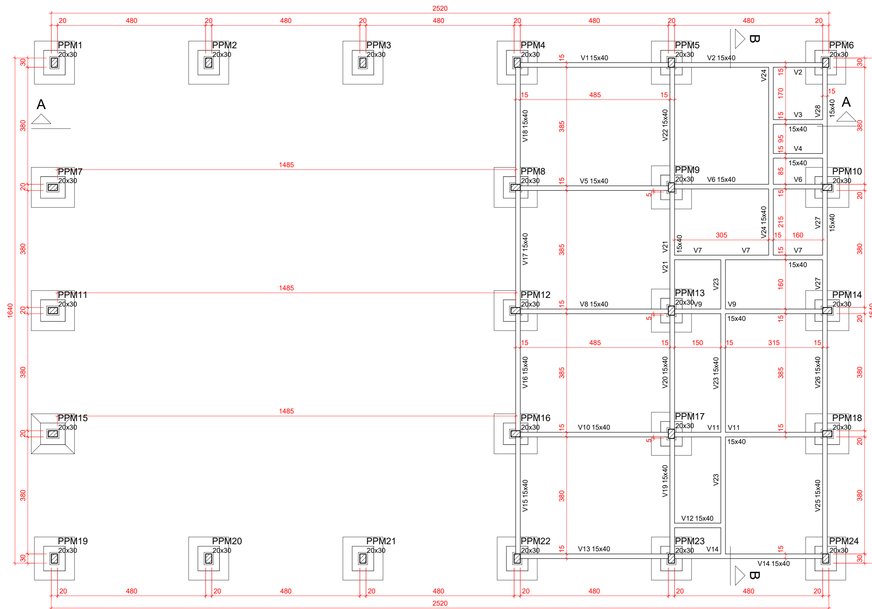
Planta de Formas do Baldrame (Nível 30)
