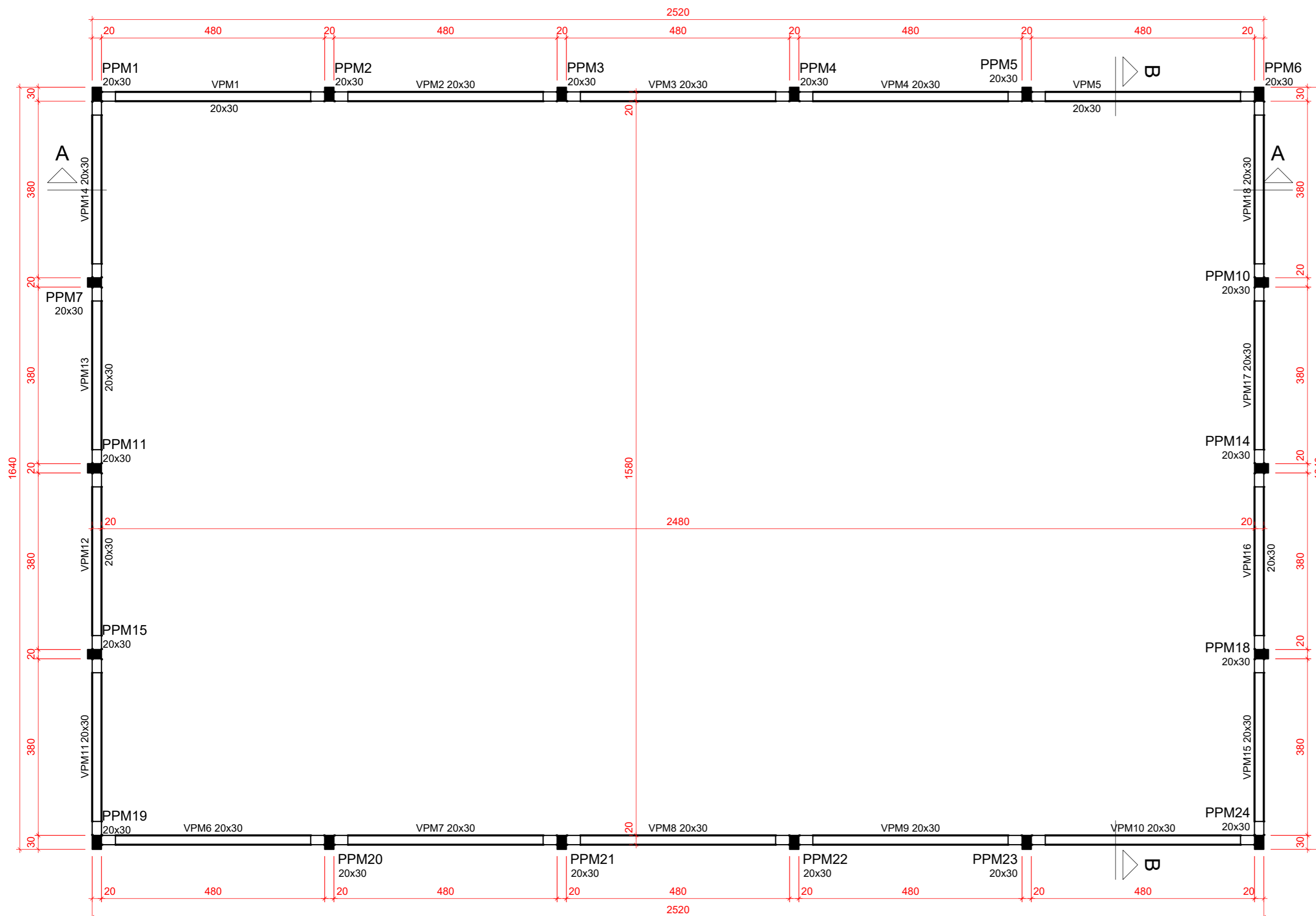
Planta de Formas da Cobertura (Nível 550)
