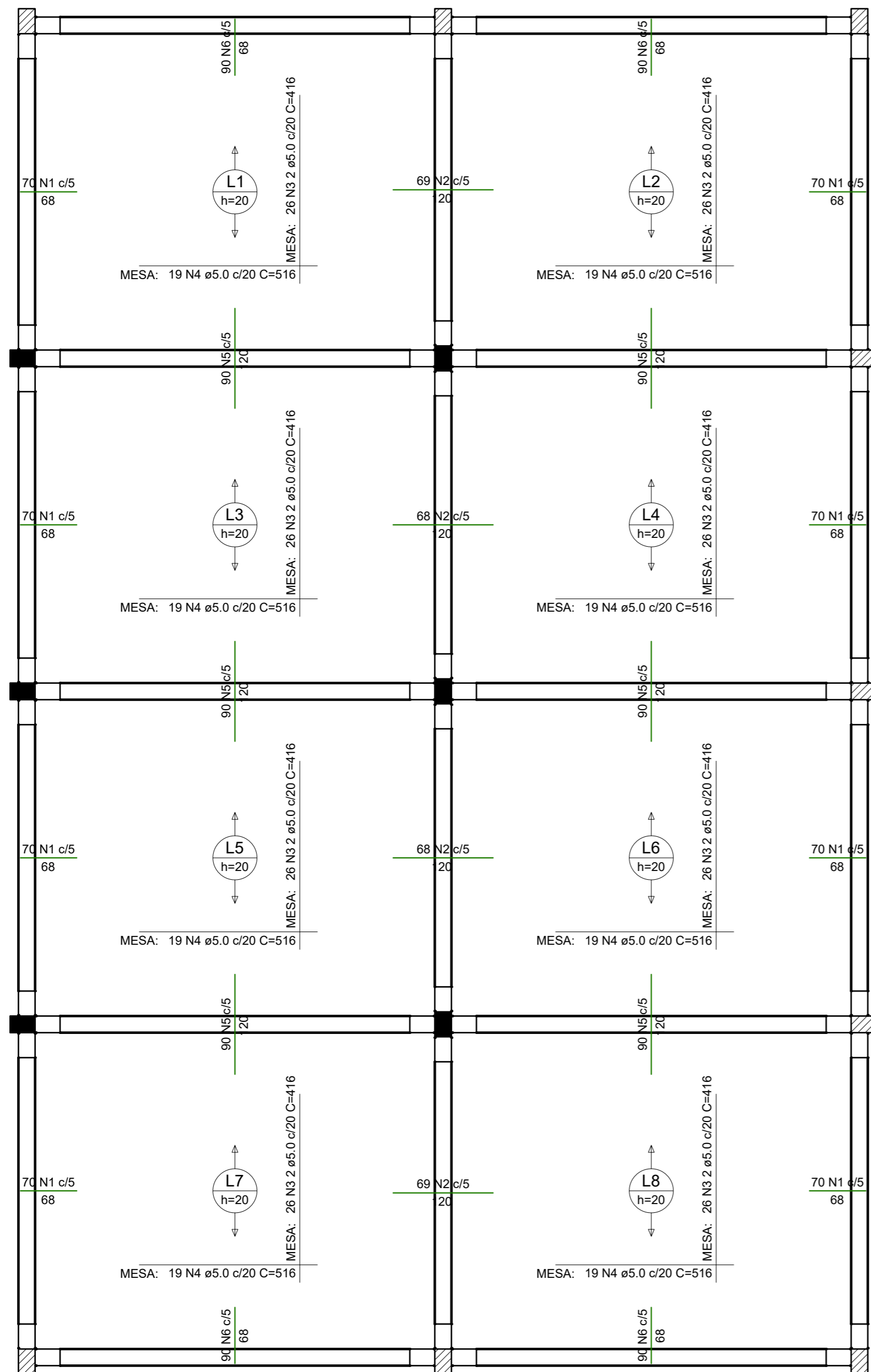
Armação das lajes do Mezanino
