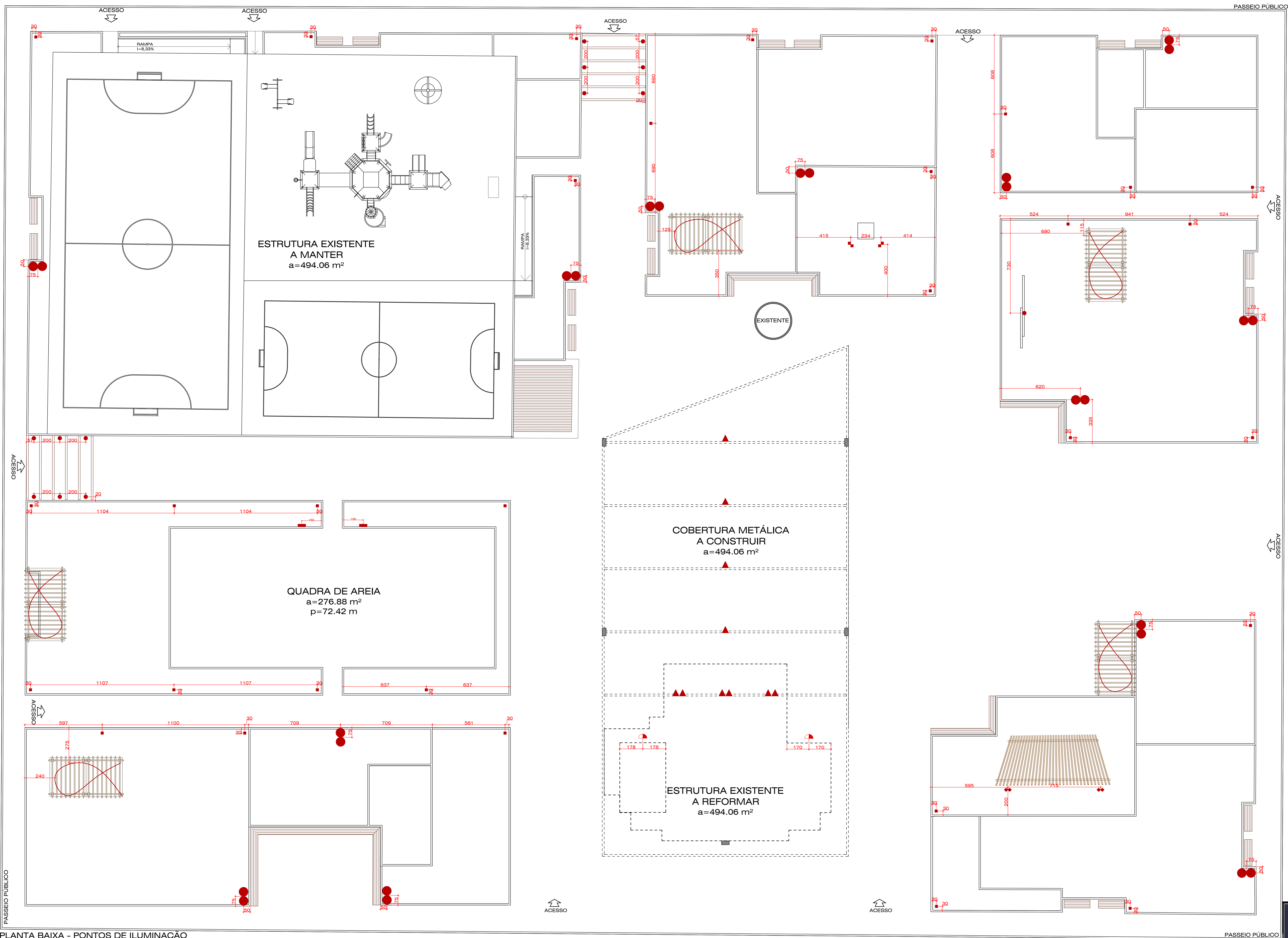
PLANTA BAIXA - PONTOS DE ILUMINAÇÃO ESC - 1:125
