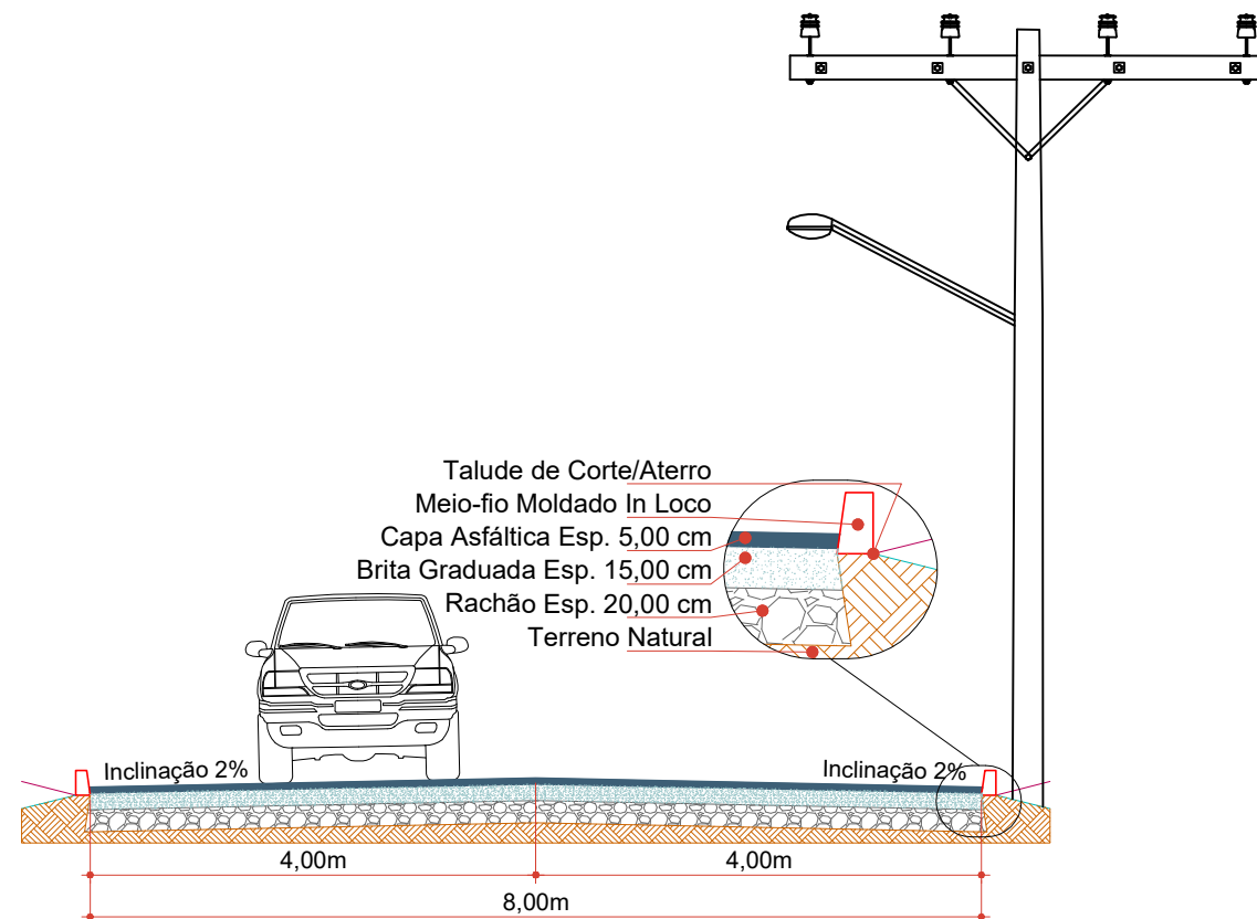
Seção Transversal Escala: 1/75
