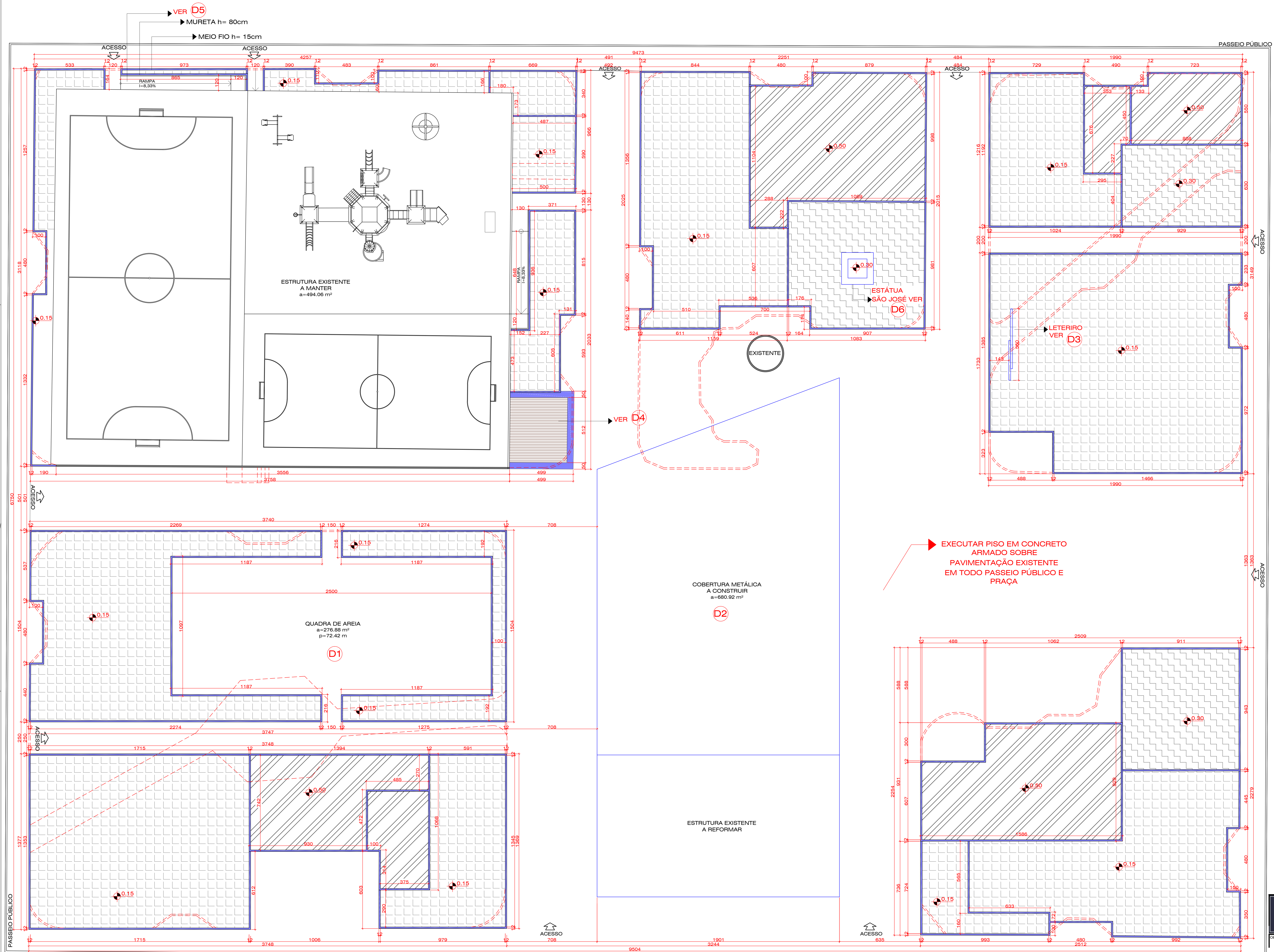
PLANTA BAIXA - A DEMOLIR E A CONSTRUIR ESC - 1:100
