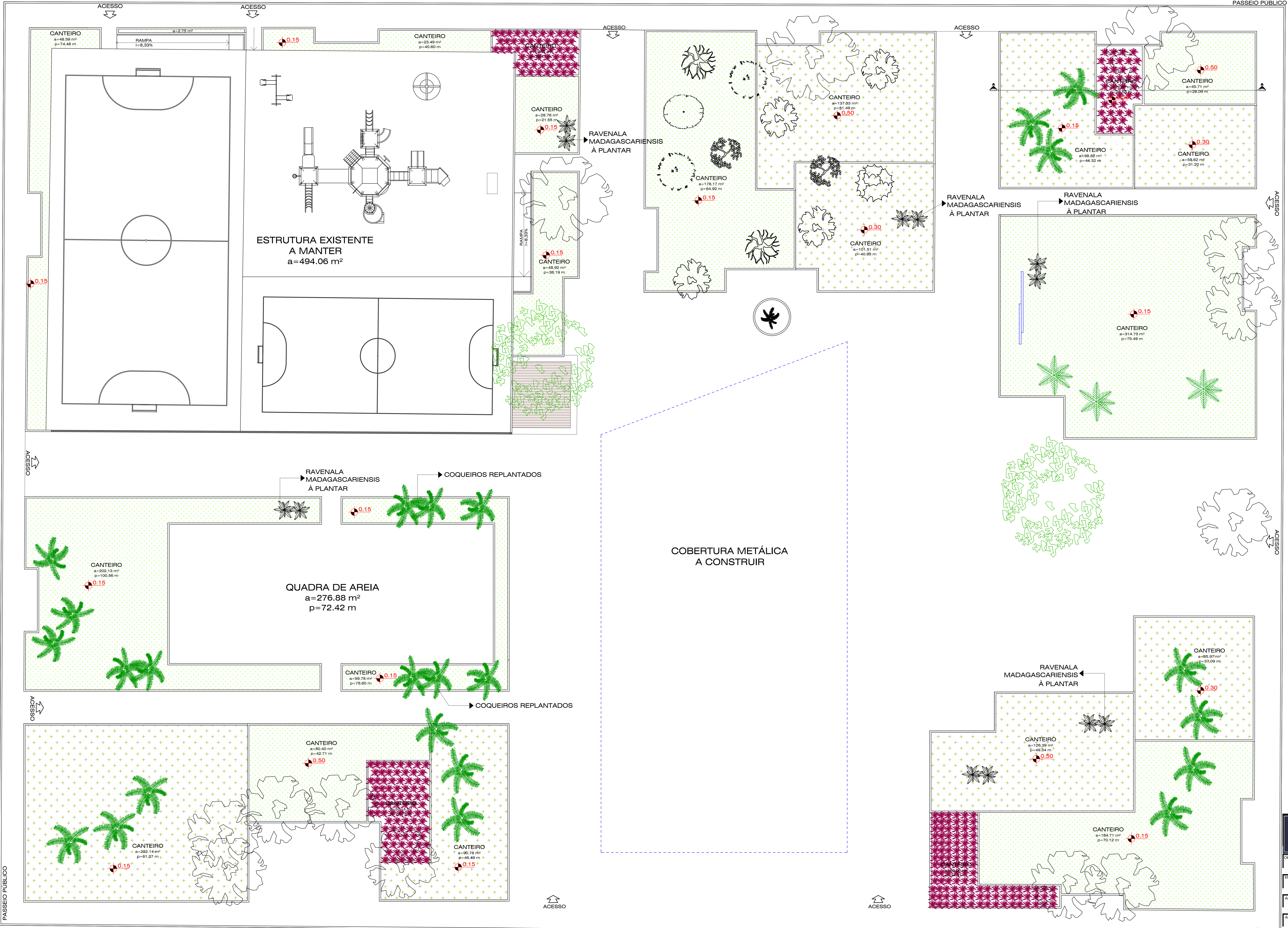
PLANTA BAIXA - CANTEIROS E PAISAGISMO ESC - 1:125
