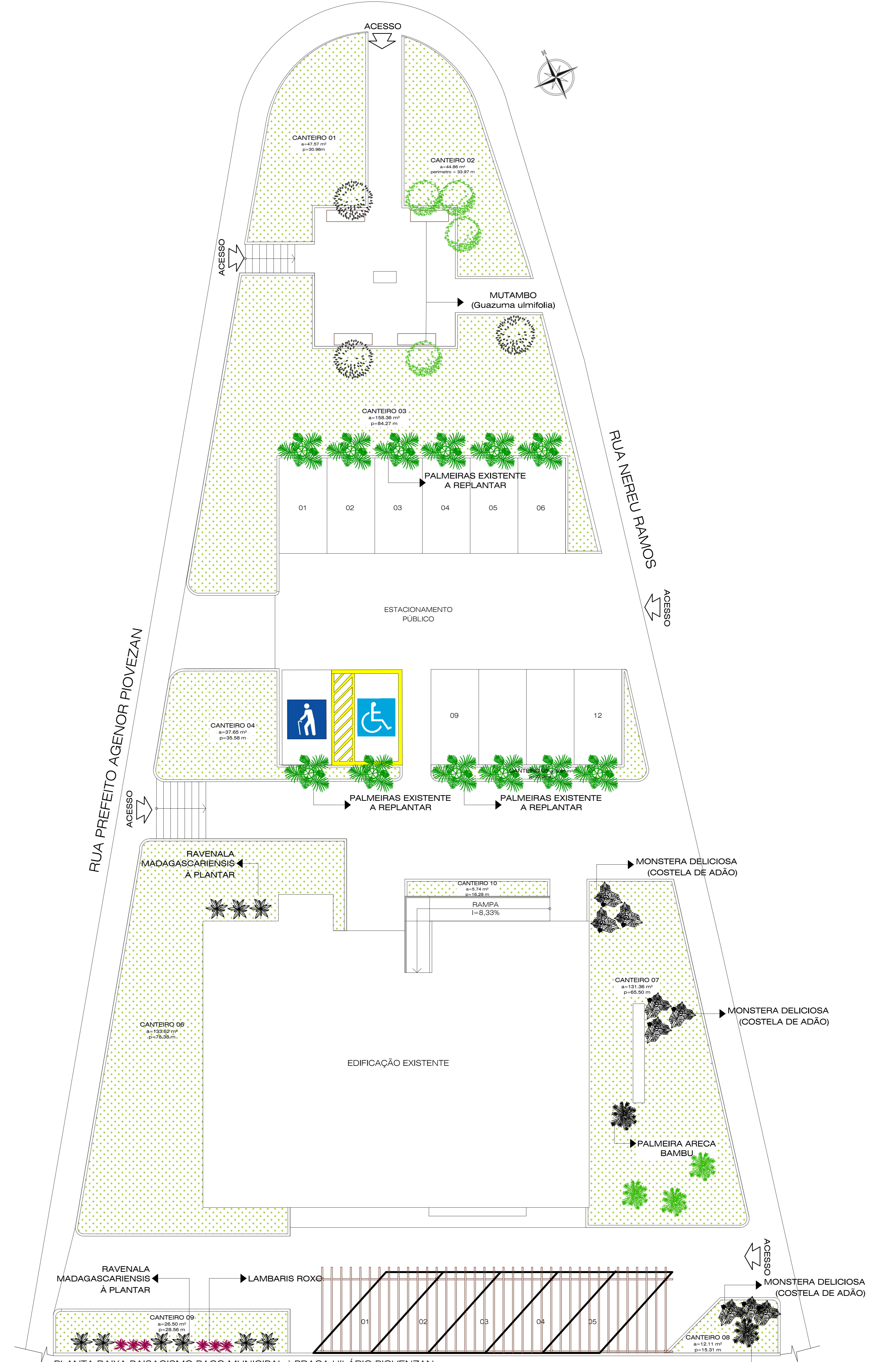
PLANTA BAIXA PAISAGISMO PAÇO MUNICIPAL | PRAÇA HILÁRIO PIOVEZAN A - 1.670,02m² ESC - 1:125
