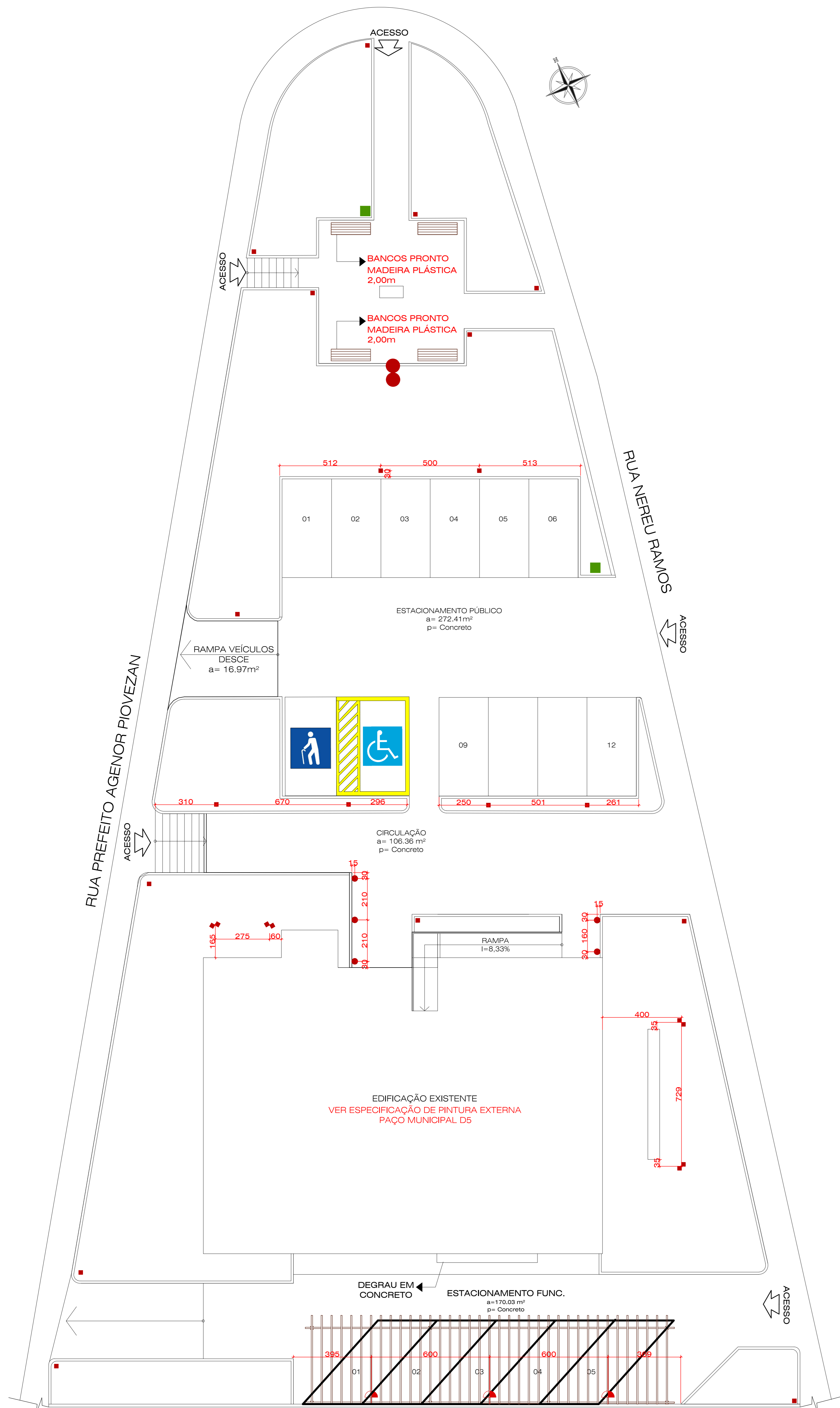
PLANTA BAIXA PAÇO MUNICIPAL | PRAÇA HILÁRIO PIOVEZAN A - 1.670,02m² ESC - 1:125
