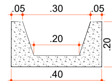
Detalhe da Canaleta Escala: 1/10
