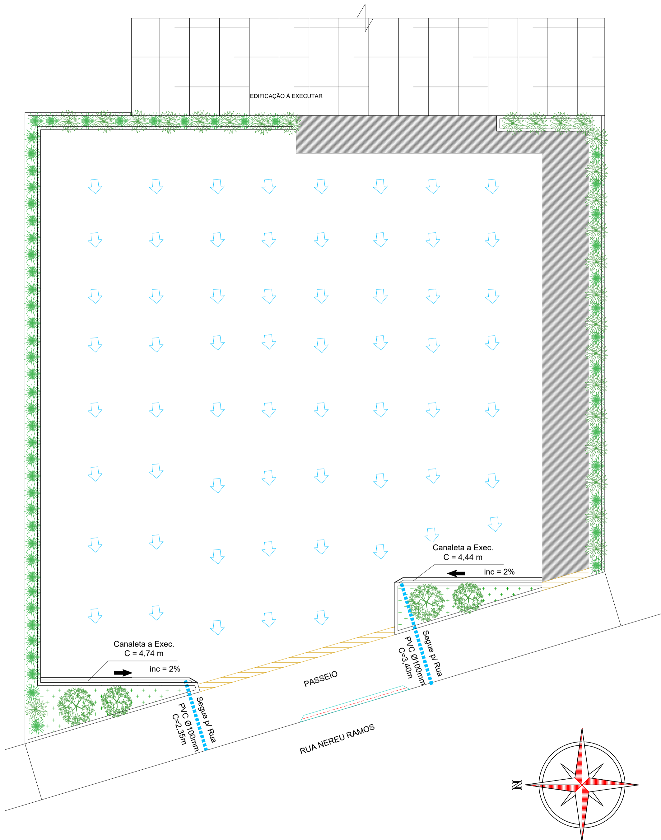
PLANTA BAIXA DRENAGEM Escala 1 : 75
