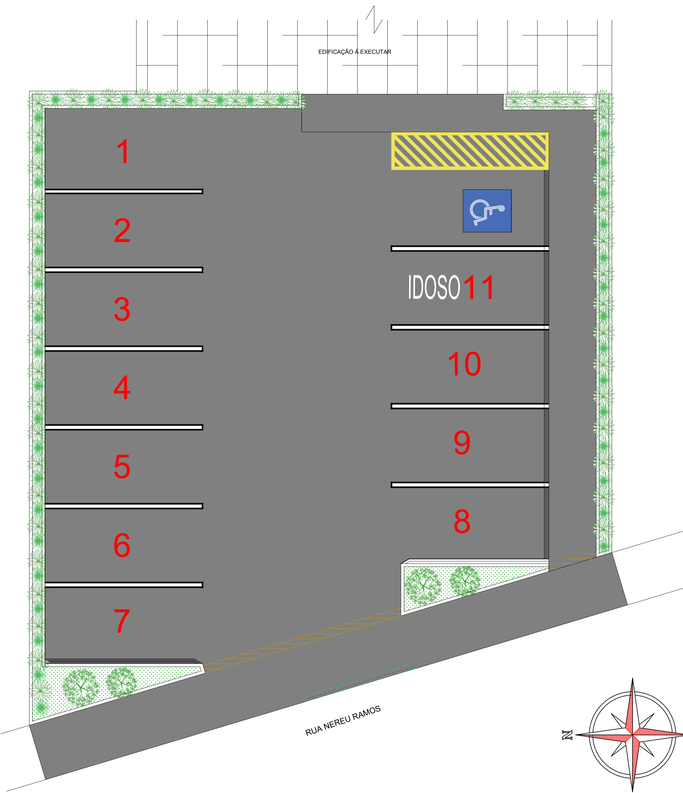
PLANTA BAIXA SINALIZAÇÃO Escala: 1:75
